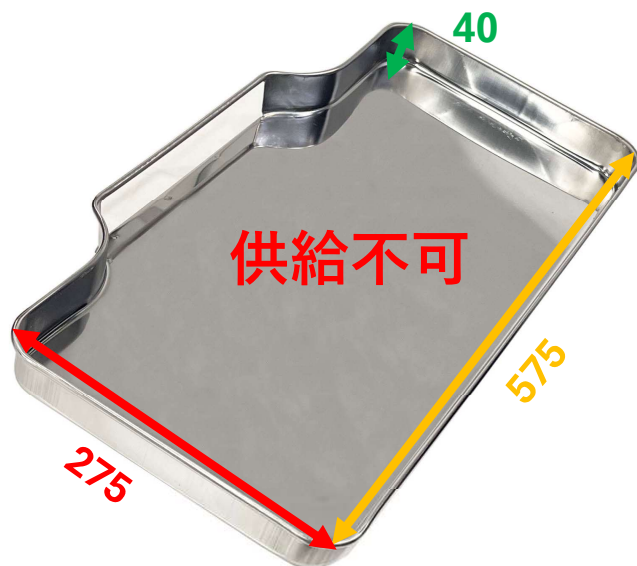
旧型油切本体
